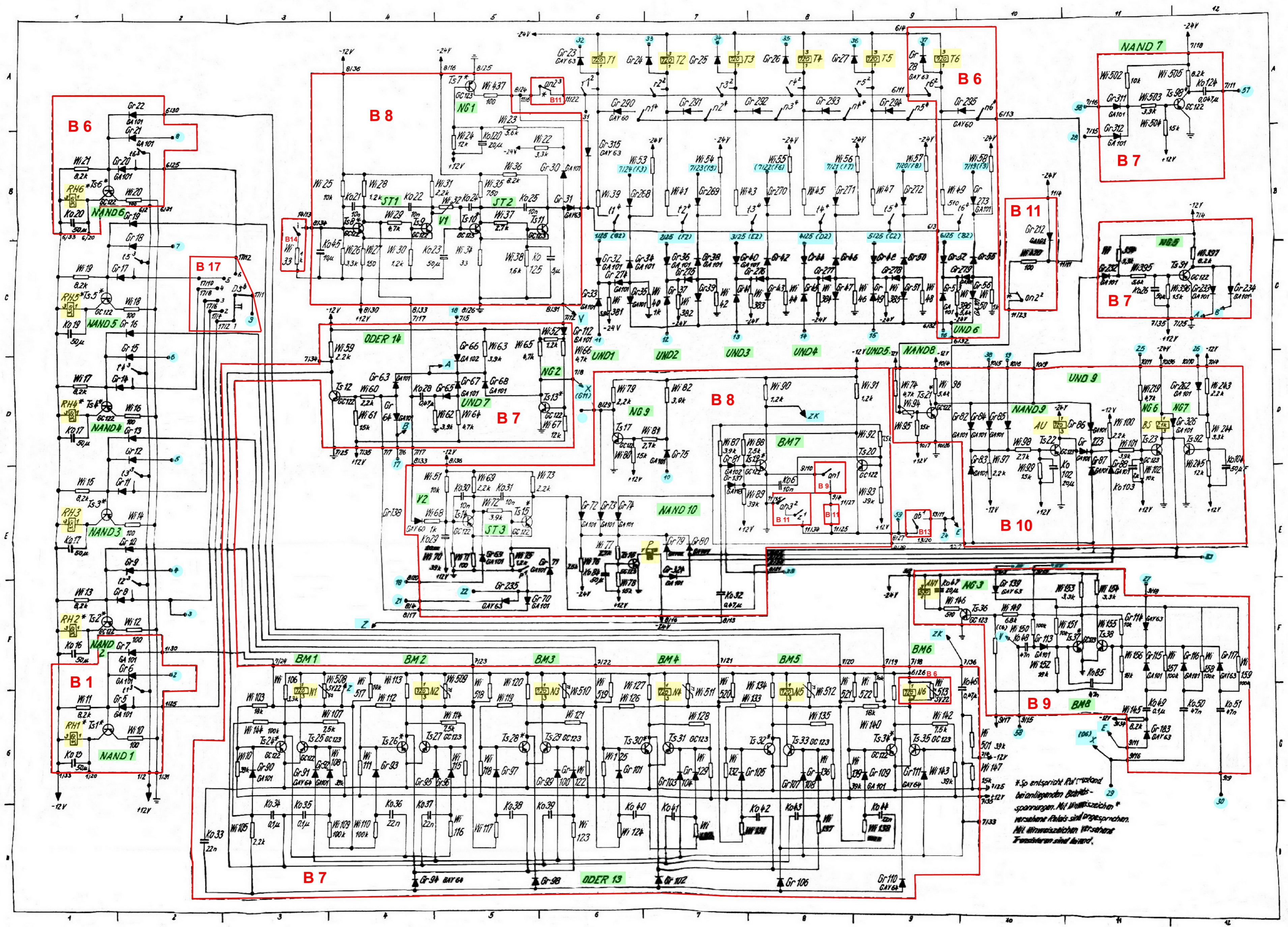
Beilage 13 Nebenstellenanlage TE 1/5/1-68: Stromlaufplan
