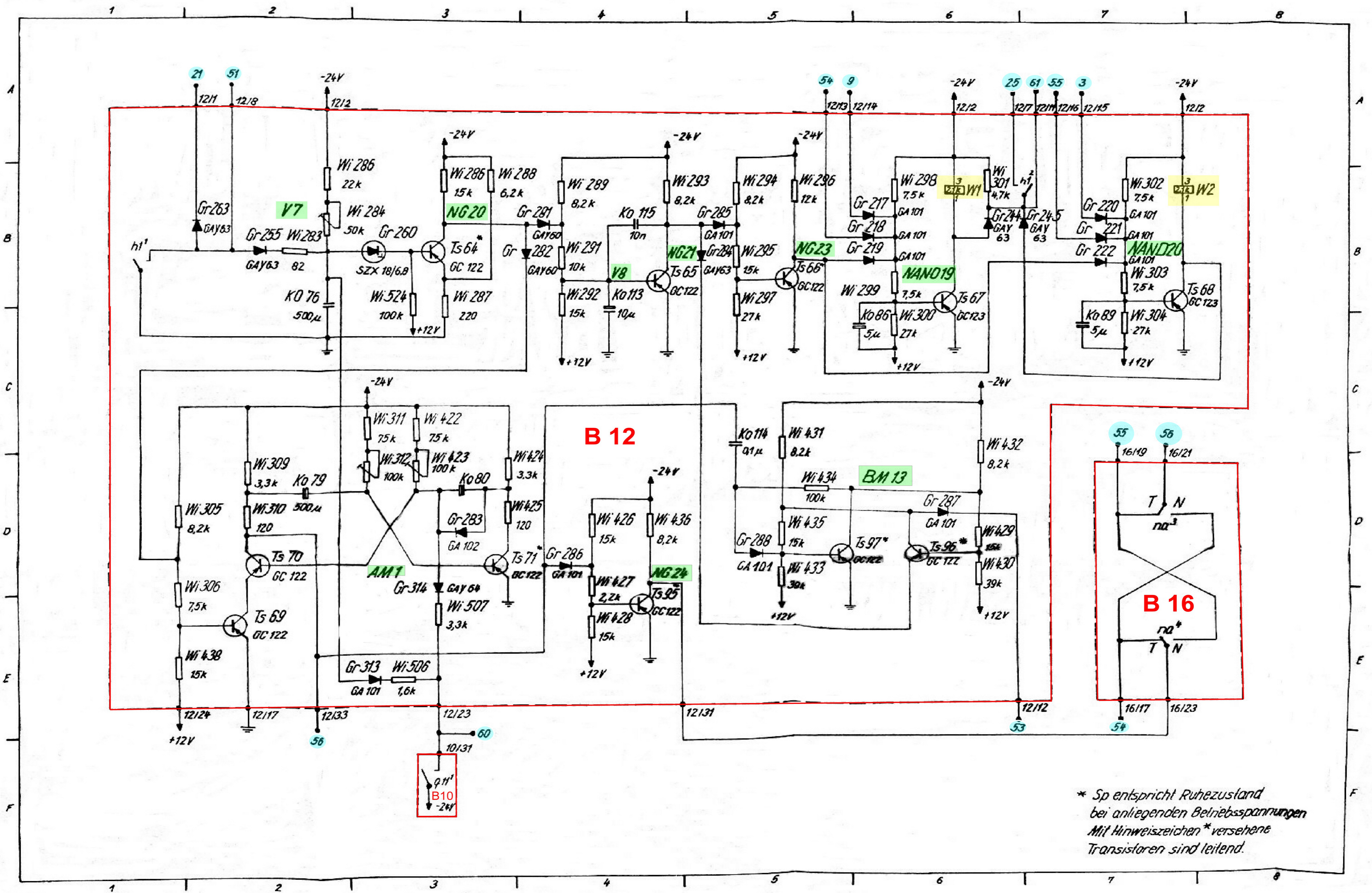
Beilage 16 Nebenstellenanlage TE 1/5/1-68; Stromlaufplan
