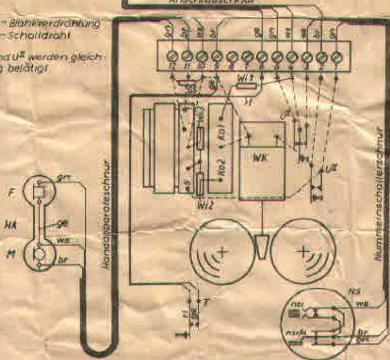
Anschlußschrur
