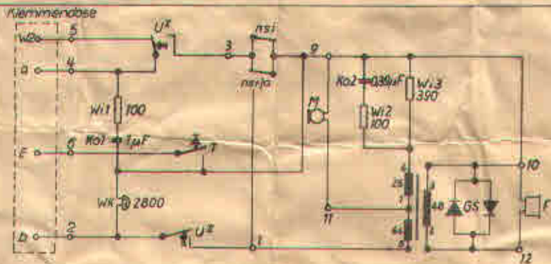
Klemmendose
